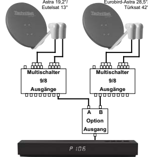
Beispiel 3: 4 Satelliten (Quattro-LNBs) Astra 19,2° Eutelsat 13° Eurobird-Astra 28,5° Türksat 42°
